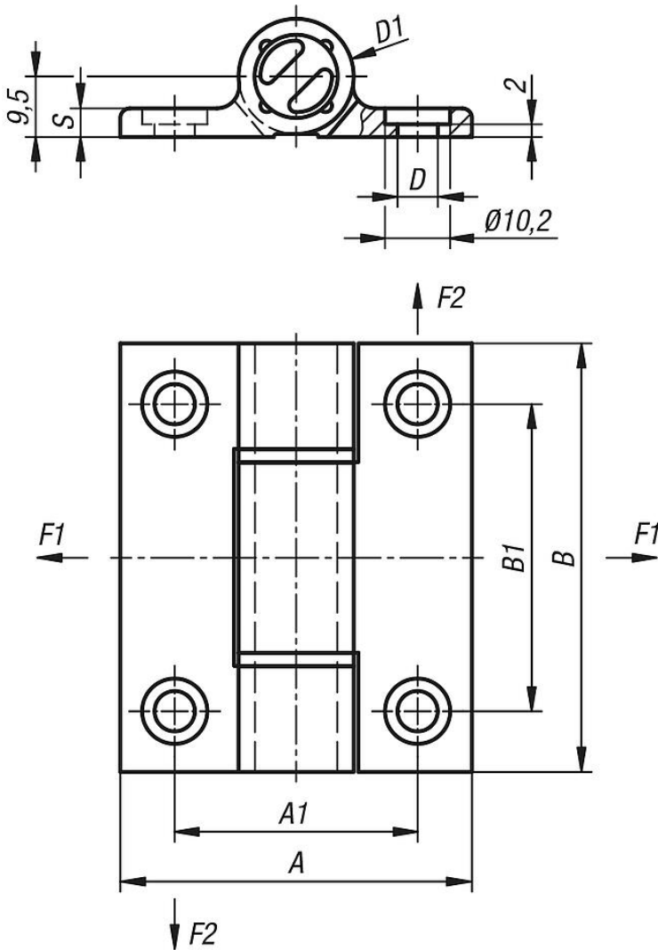
Scharniere mit Öffnungsfeder, öffnend
